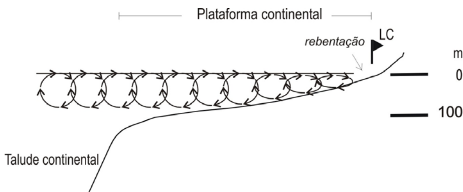
Fig. 10 – A modificação do movimento orbital com a aproximação de terra. LC - linha de costa.
