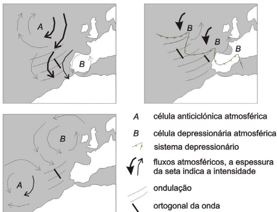
Fig. 11 – Ondulação de noroeste, gerada no bordo oriental de um anticiclone e numa situação pós-frontal.
