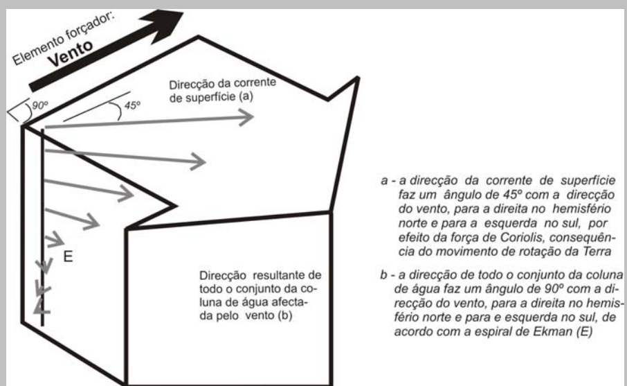
Fig. 9.1 – O transporte de Ekman. Baseada em Duxbury e Duxbury (1993).
