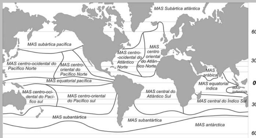
Fig. 6.1 – As massas de água superficiais oceânicas. Adaptado de Brown et al, 1993.
