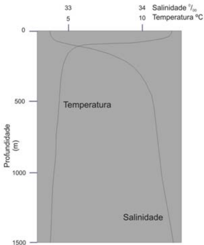
Fig. 5 – Diagrama da variação da temperatura e da salinidade com a profundidade.
