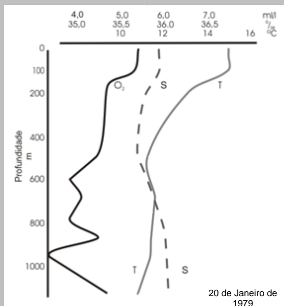
Fig. 5.1 – Variação, em profundidade, da temperatura (T), salinidade (S) e teor em oxigénio ( O_2 ) da água do oceano Atlântico, ao Largo da Figueira da Foz.
