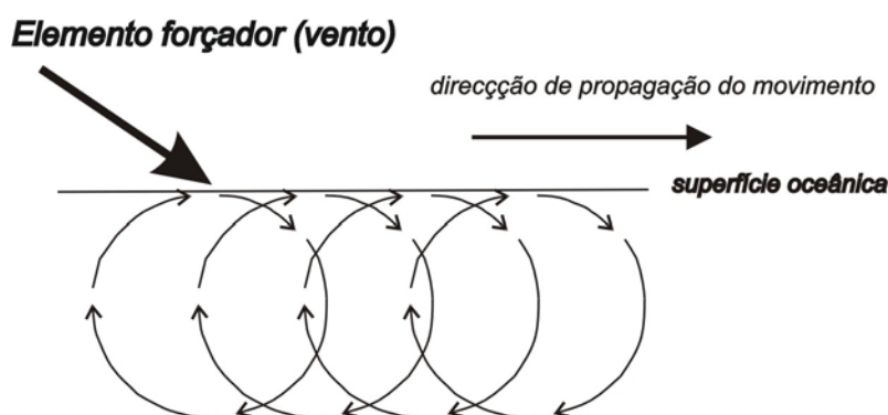
Fig. 9 – O movimento ondulatório das partículas de água criado pelo vento.
