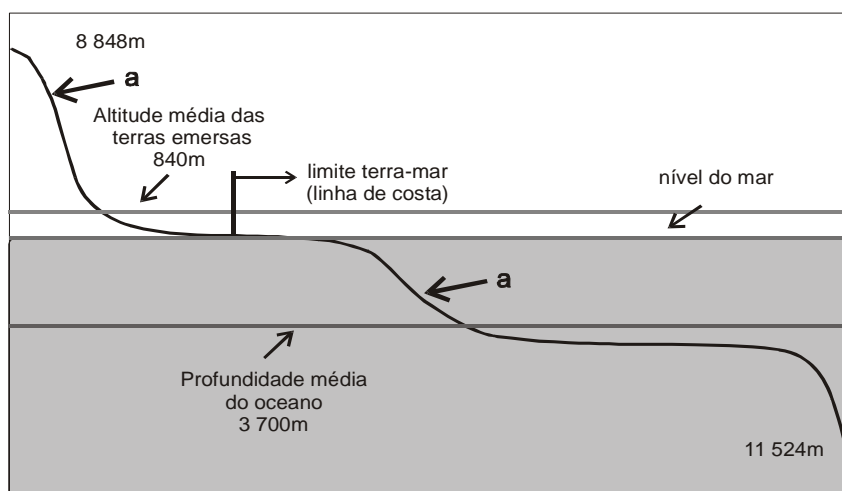
Fig. 2 – Curva hipsométrica global (a).
